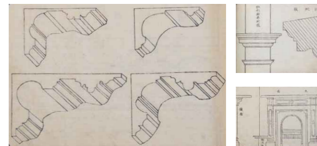
「和洋左官雛形」 泉幸次郎著／鈴木光蔵(1902年) Drawing Manual for Japan and Western Mix Plaster Design 雛形本の形式をもち、「西洋造」の立面を描き、天井蛇腹の線形や持ち送り、様々なマンテルピースの見本例を図示。一方で後半では、伝統的な土蔵や土堀、江戸時代以来の絵様の図解もあわせて掲載されています。
